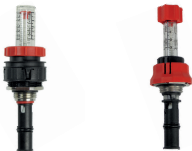
Débitmètre (Collecteur en acier inox. 1")
